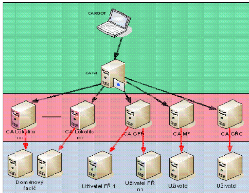
Obrázek 2 - schéma navrhovaného uspořádání cert. autorit
