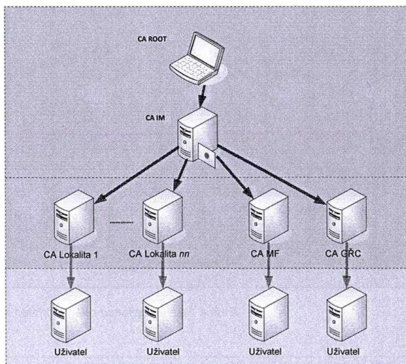
Obrázek 1 - schéma stávajícího uspořádání cert. autorit
