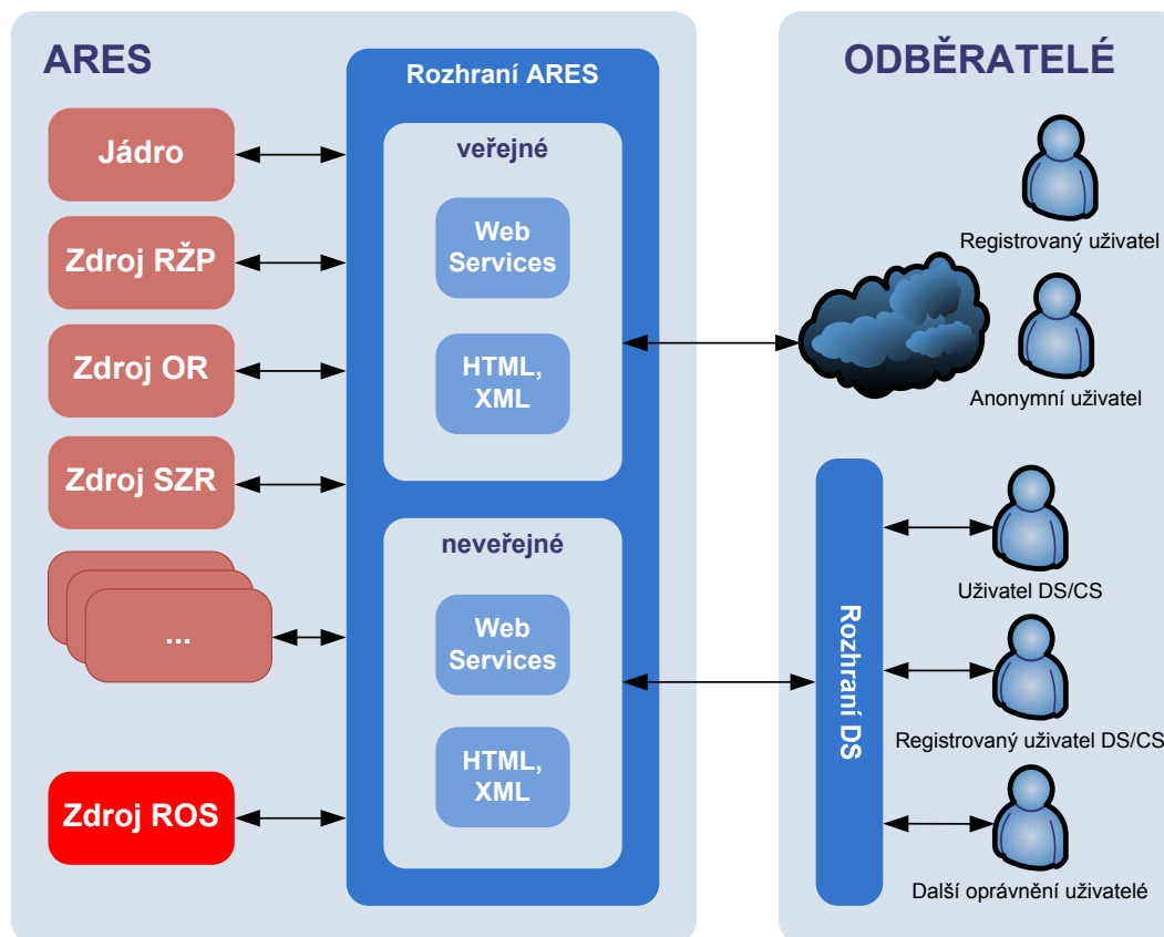
Obrázek 2 – ARES – blokové schéma
