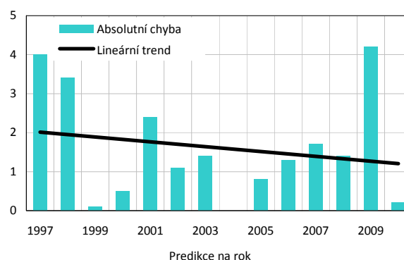
Graf 8: MAE v horizontu 18 měsíců
